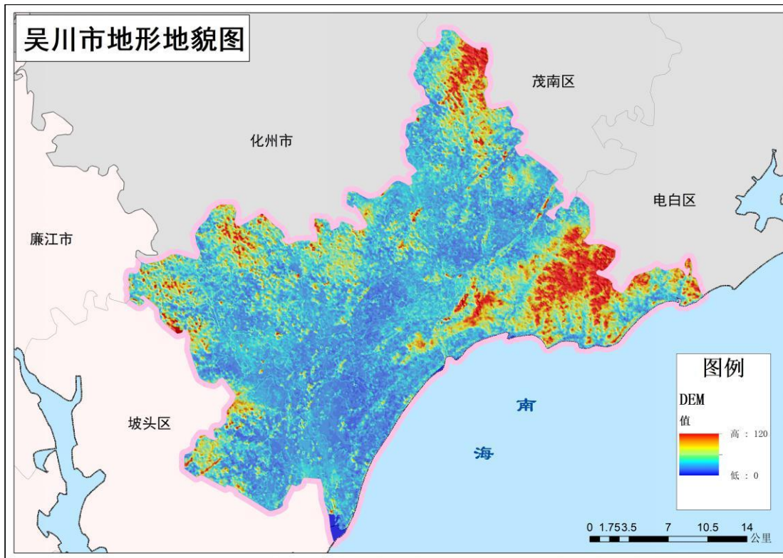
图 1-3 吴川市地形地貌
