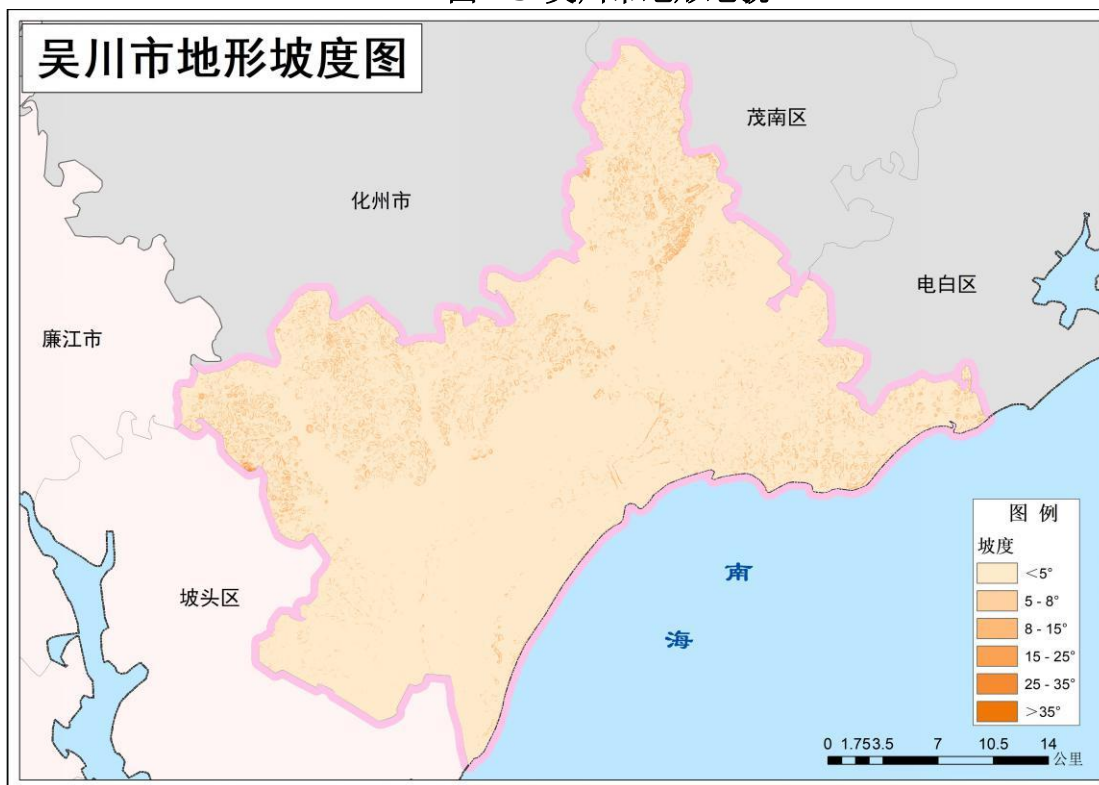
图 1-4 吴川市坡度分级图
