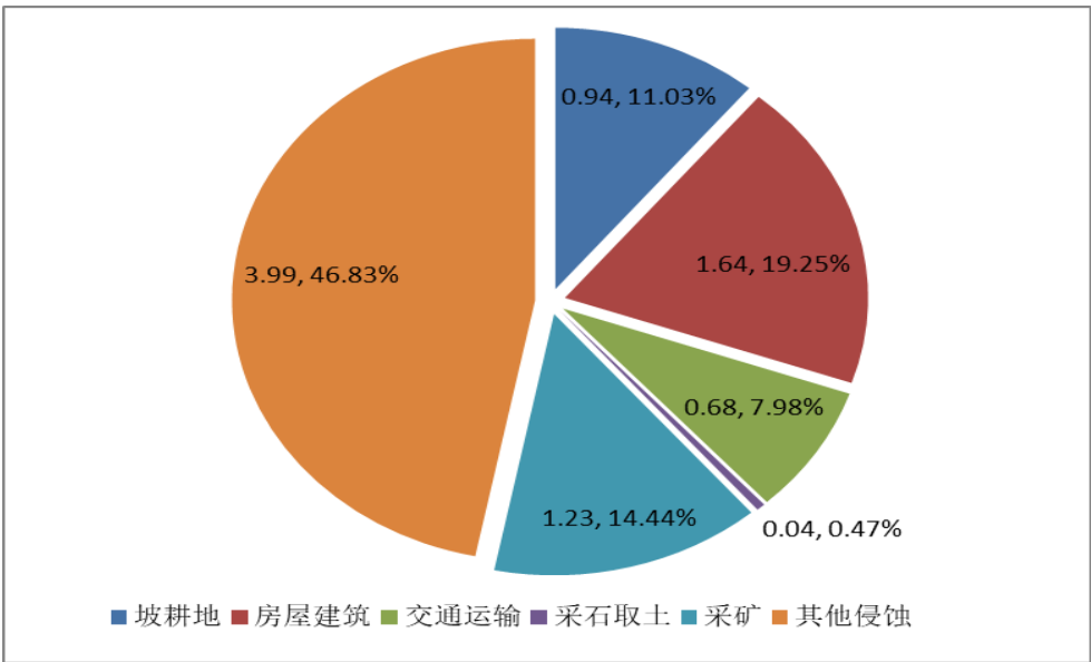
图 2-1 吴川市人为侵蚀各强度占比
