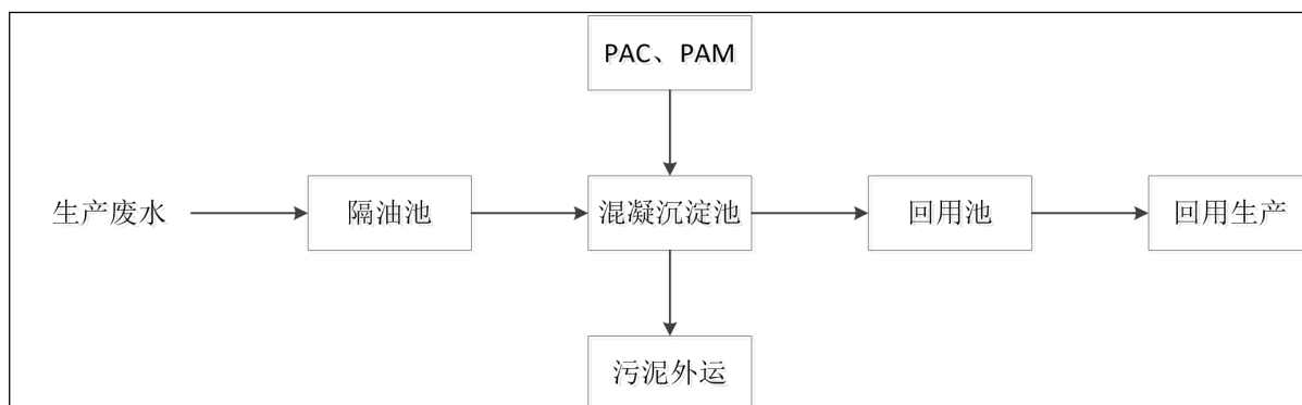
图 4-1 项目污水处理流程图
