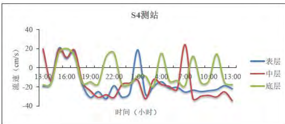
图 3-10 S4 测站实测海流流速过程图
