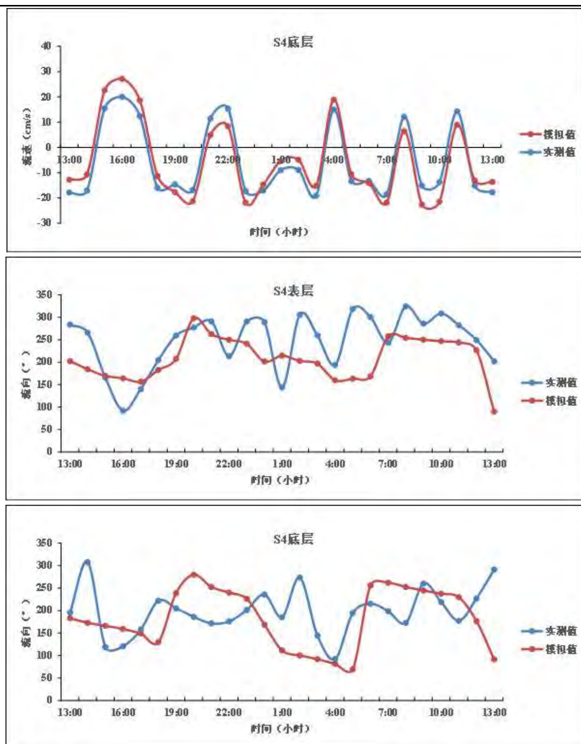
图 4-3 S4 测站表底层流速流向
