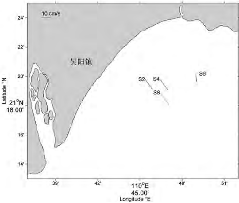
图 3-19 测站表层余流
