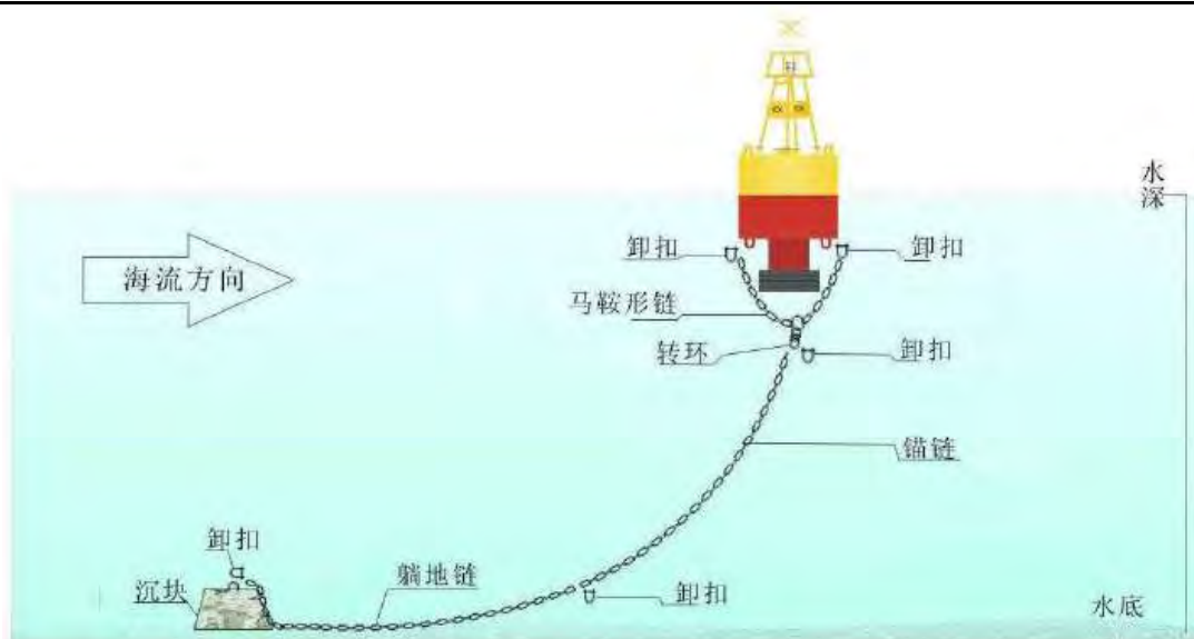
图 2-5 浮标效果图
