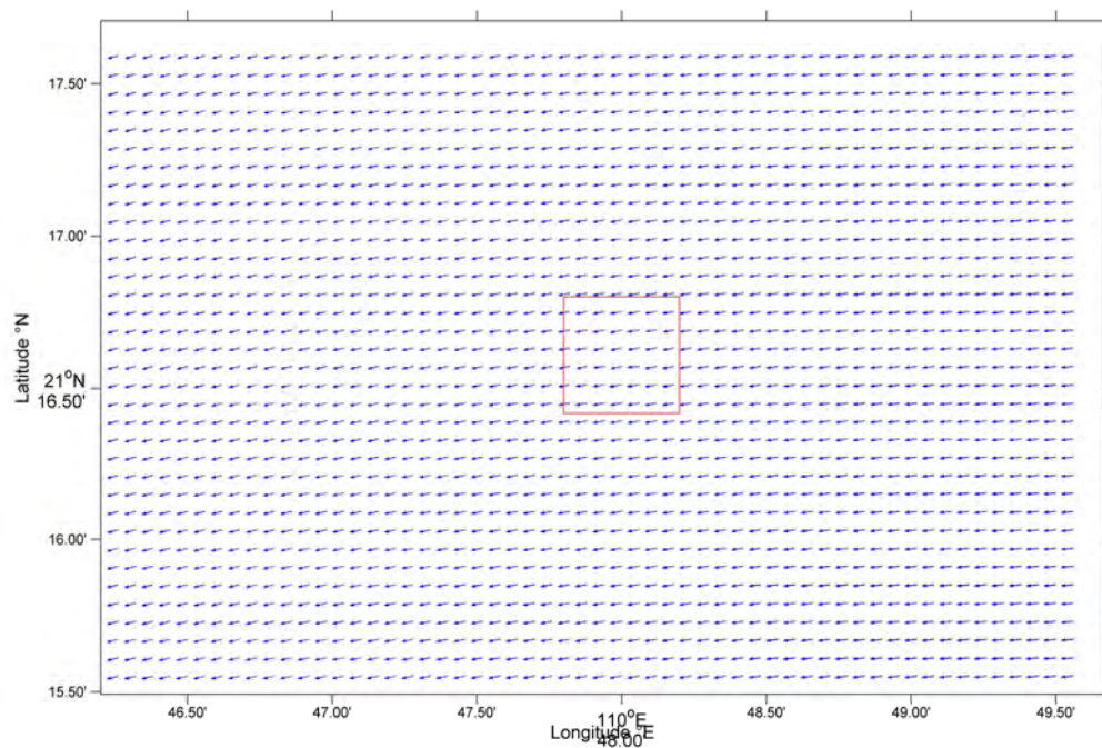
图 4-11 吴川博茂人工鱼礁建成后底层涨急流场
