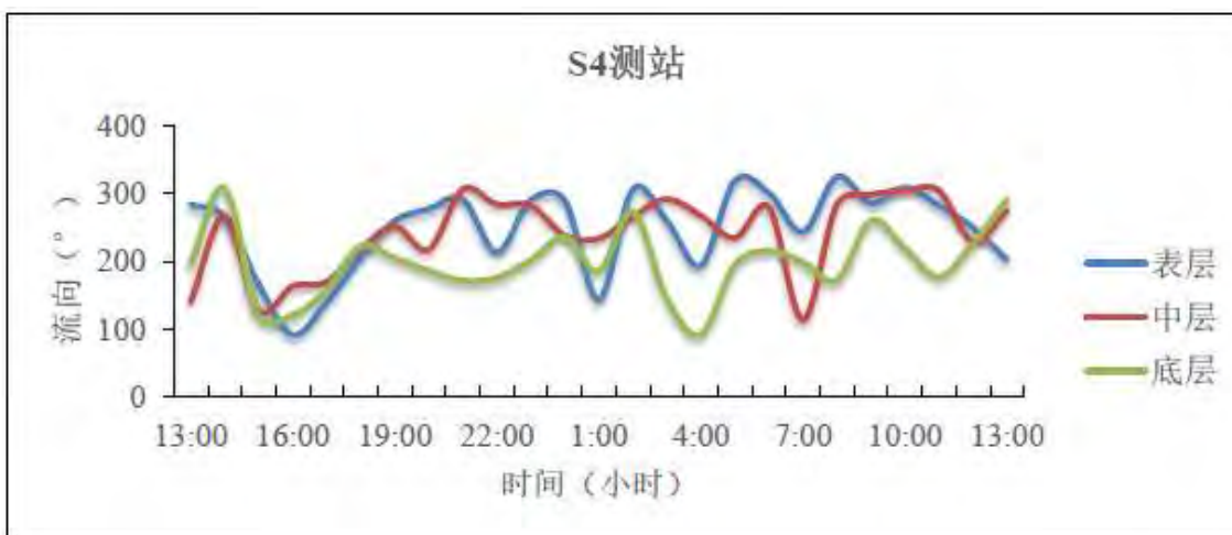
图 3-11 S4 测站实测海流流向过程图
