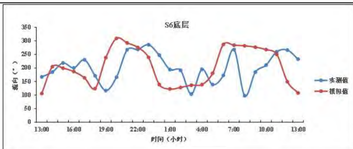
图 4-4 S6 测站表底层流速流向
