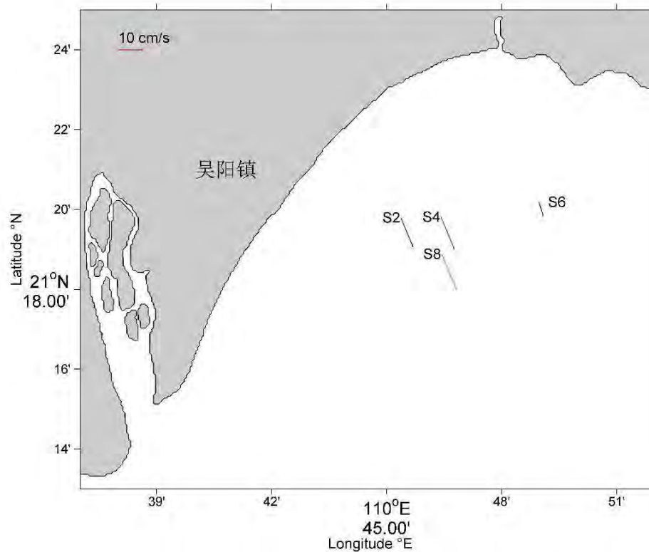
图 3-20 测站中层余流
