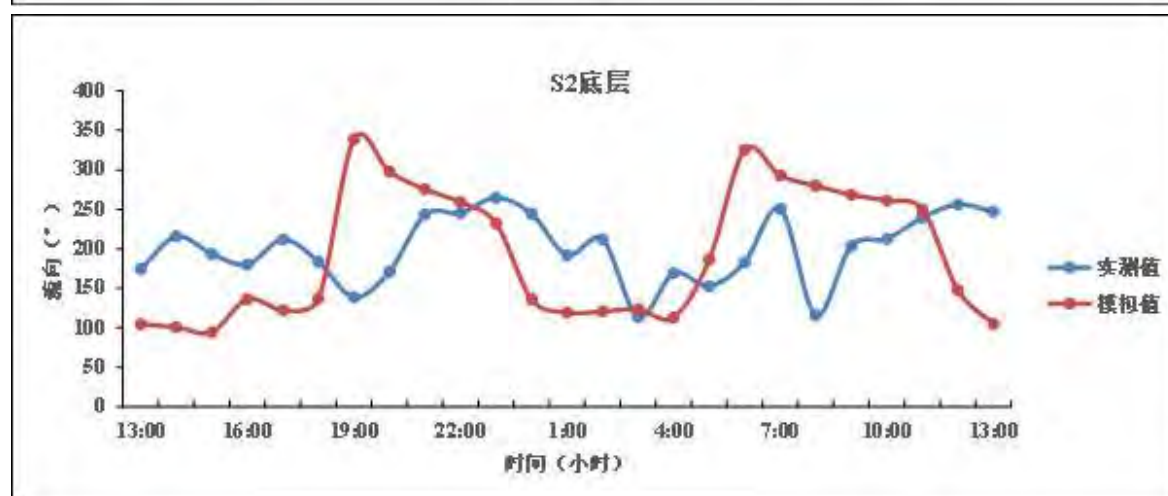
图 4-2 S2 测站表底层流速流向
