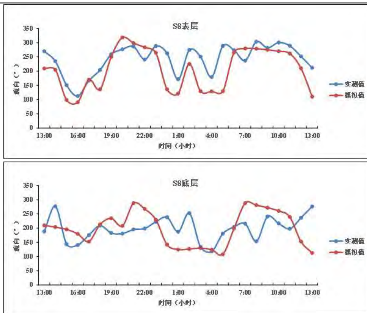
图 4-5 S8 测站表底层流速流向
