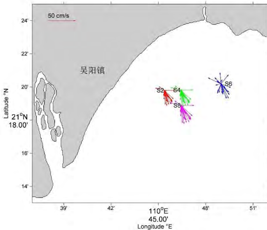
图 3-17 测站中层实测海流玫瑰图
