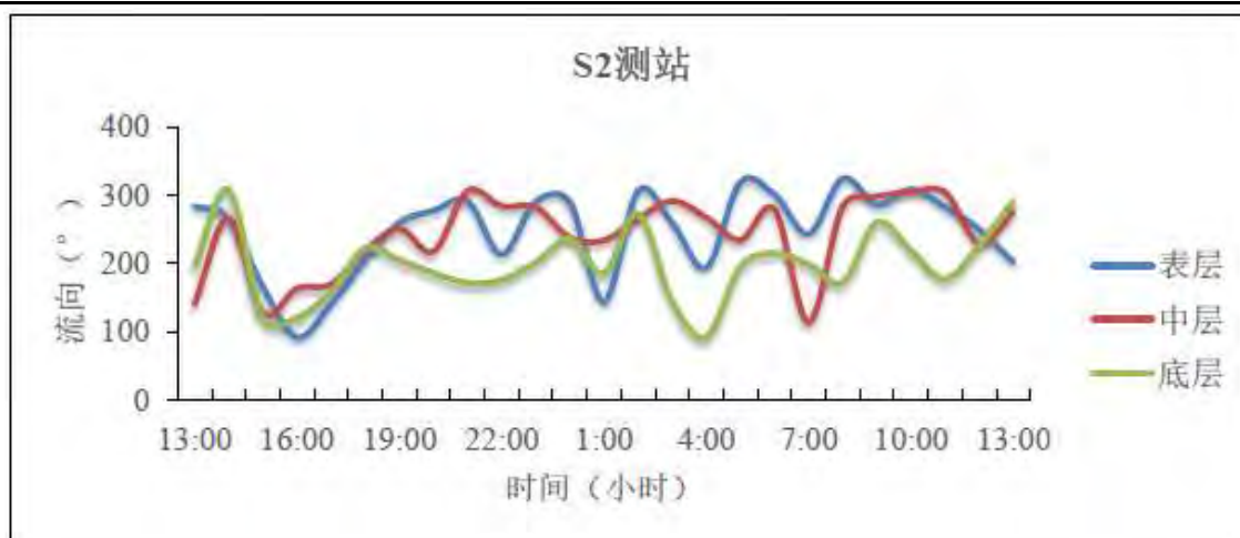
图 3-9 S2 测站实测海流流向过程图
