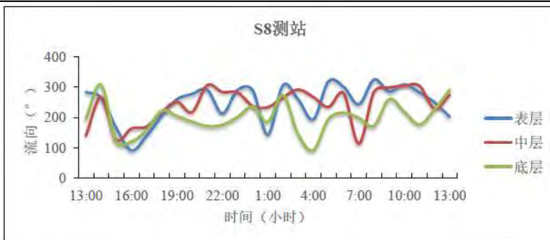
图 3-15 S8 测站实测海流流向过程图
