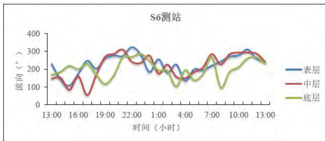
图 3-13 S6 测站实测海流流向过程图
