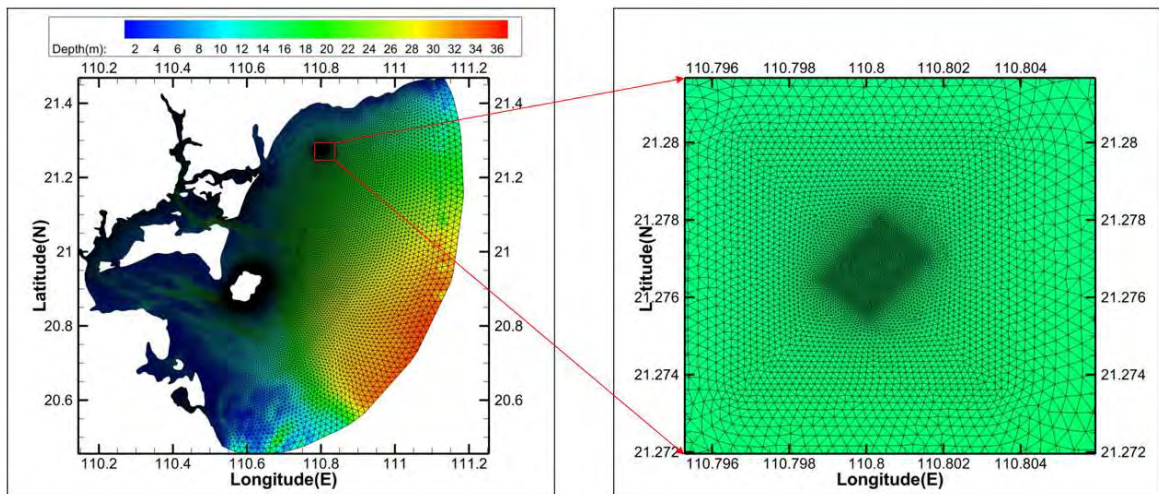
图 4-1 计算区域网格水深和人工鱼礁区局部细节网格水深
