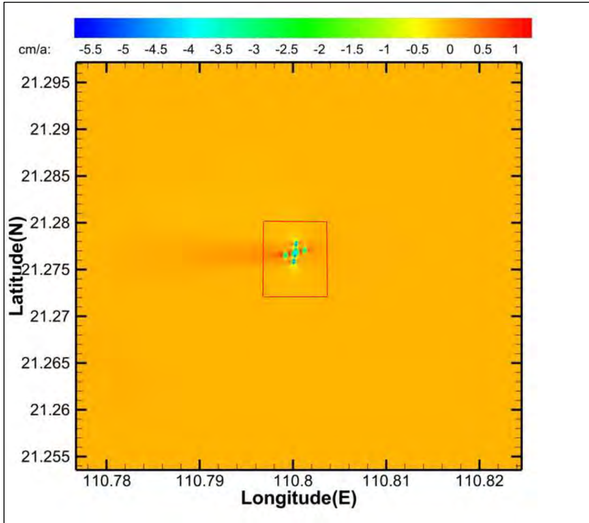
图 4-14 人工鱼礁建成后泥沙冲淤分布情况（单位：cm/a）
