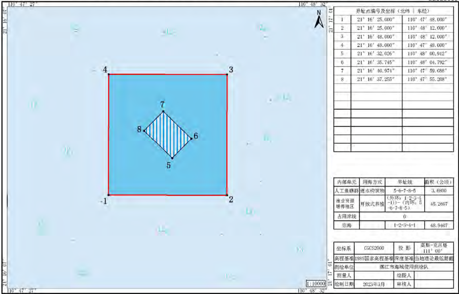
广东省吴川博茂海域国家级海洋牧场示范区人工鱼礁建设项目宗海界址图
