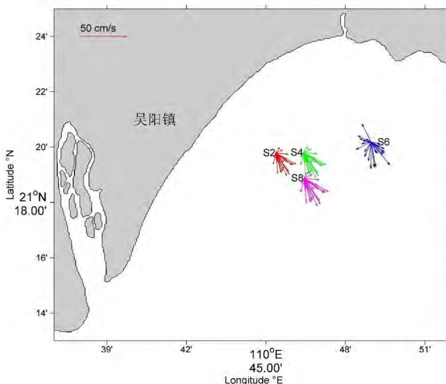
图 3-16 测站表层实测海流玫瑰图
