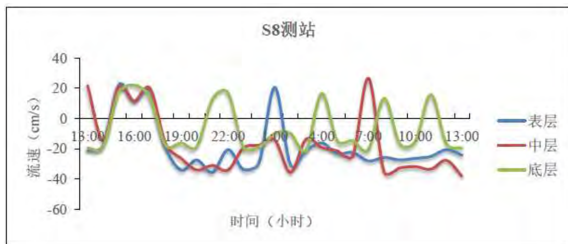
图 3-14 S8 测站实测海流流速过程图
