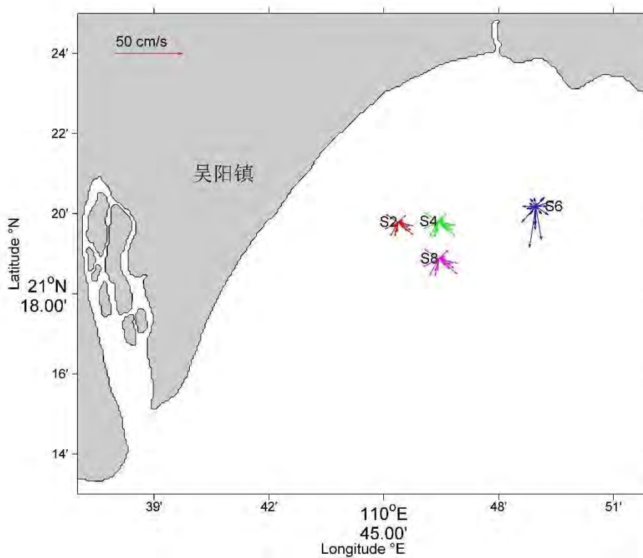
图 3-18 测站底层实测海流玫瑰图
