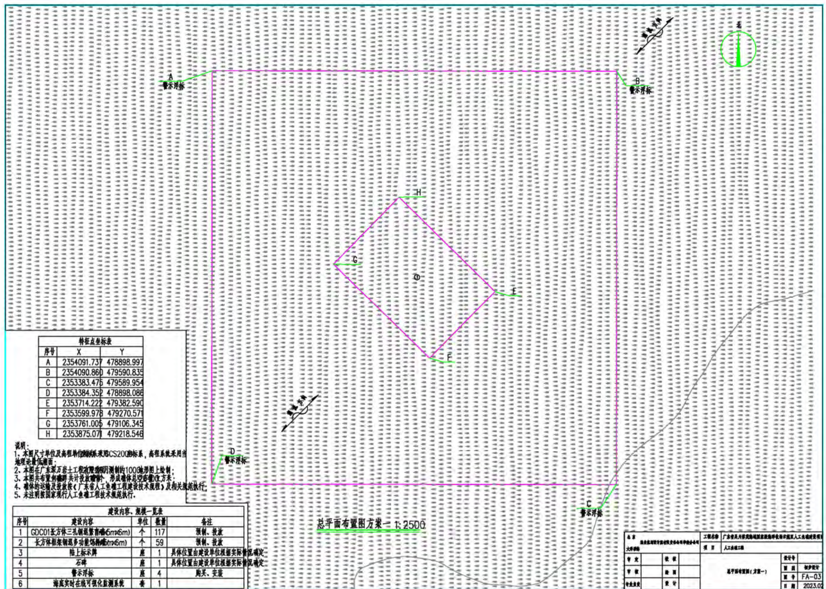
附图 2 总平面布置图
