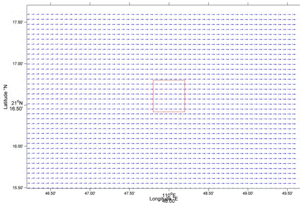
图 4-9 吴川博茂人工鱼礁建设前底层落急流场
