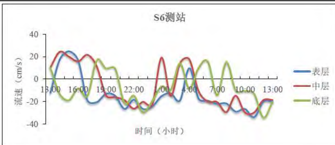
图 3-12 S6 测站实测海流流速过程图
