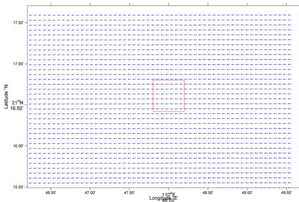
图 4-10 吴川博茂人工鱼礁建成后表层涨急流场
